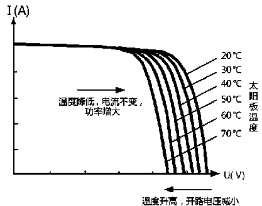
图 1-4 电池板输出特性与温度的关系
